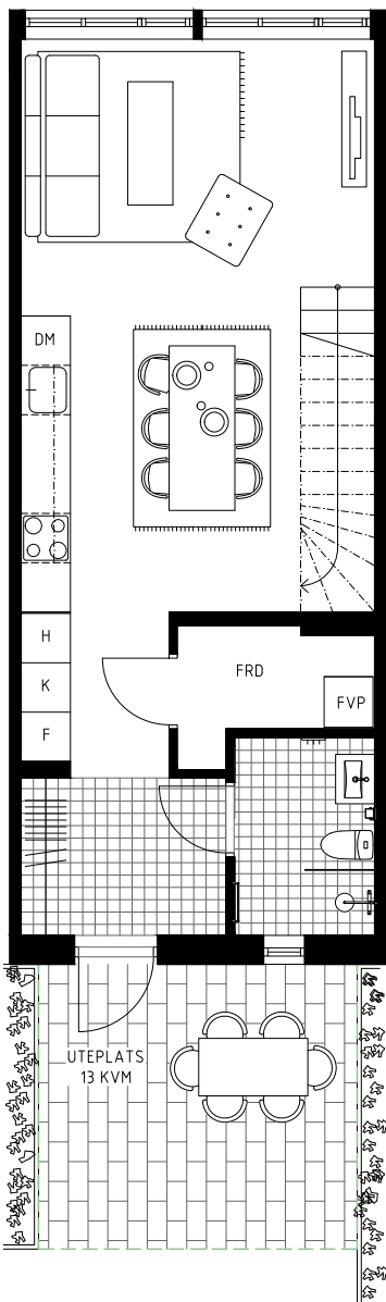
ENTRÉPLAN
