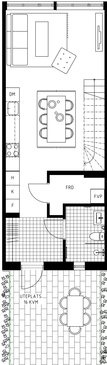
ENTRÉPLAN
